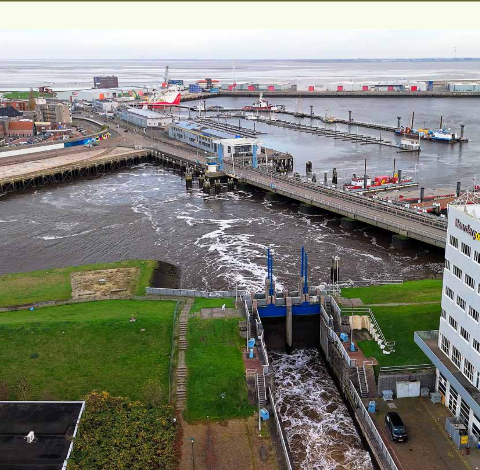
Spuisluis Delfzijl
