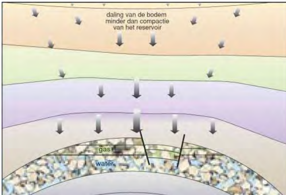
Figuur. 3.1 Ontstaan van de bodemdalingsskom door compactie van het reservoir [5]
