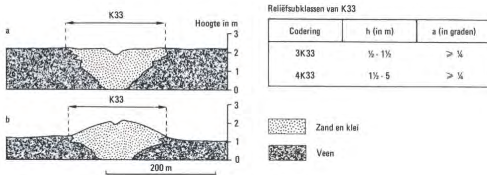
Figuur 4.6 Schematische doorsnede van een getij-inversierug (K33) voor (a) en na (b) de klink [10].
