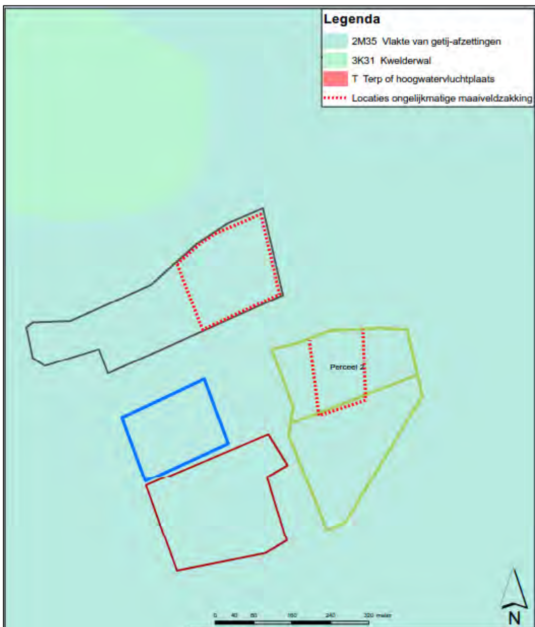
Figuur 5.5 Geomorfologische kaart (volledige kaart is opgenomen in bijlage 7).
